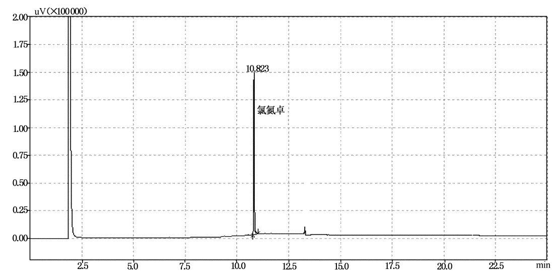
图 B.1 氯氮卓气相色谱图
